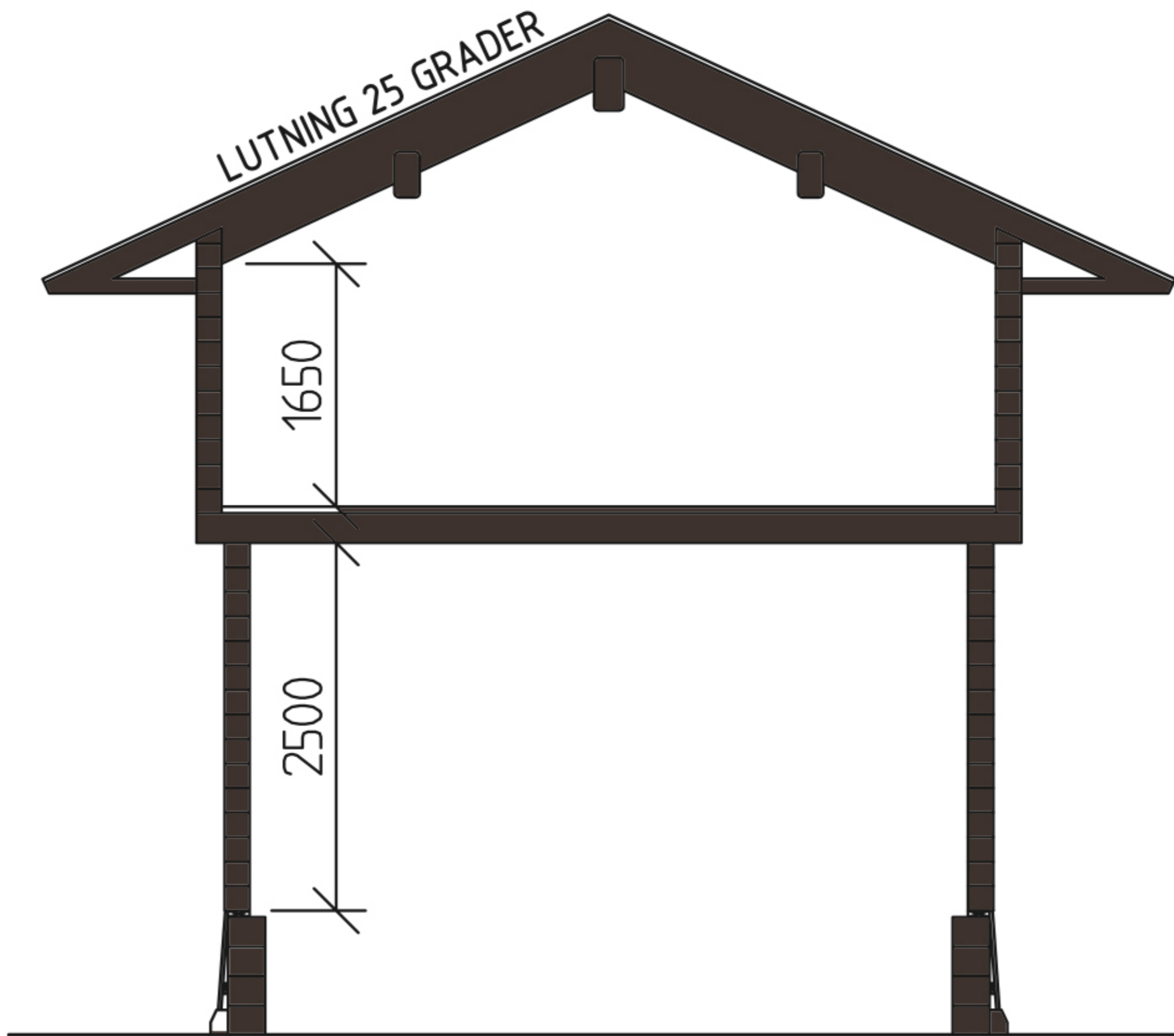
PRINCIPSEKTION
