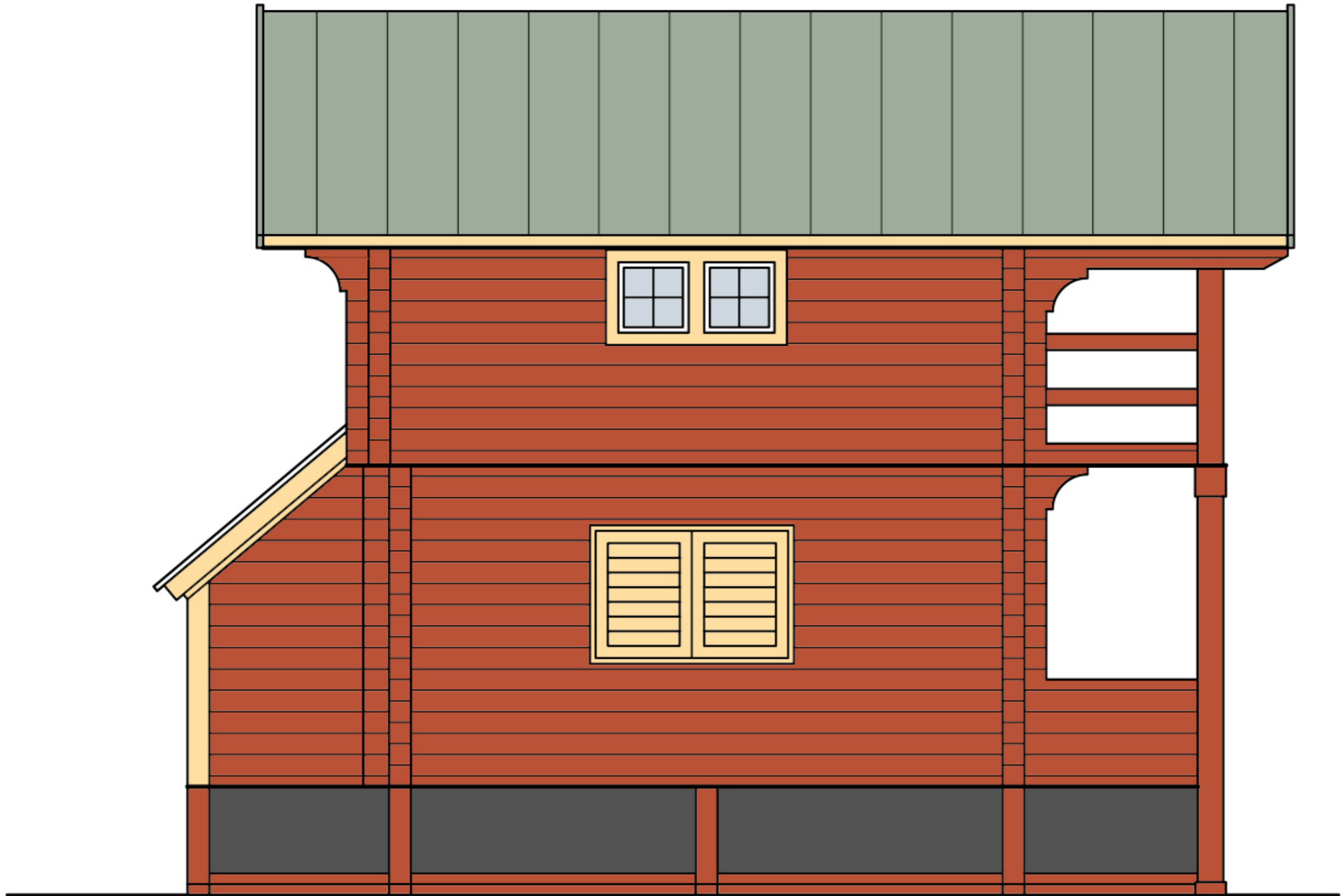
SIDOFASAD
