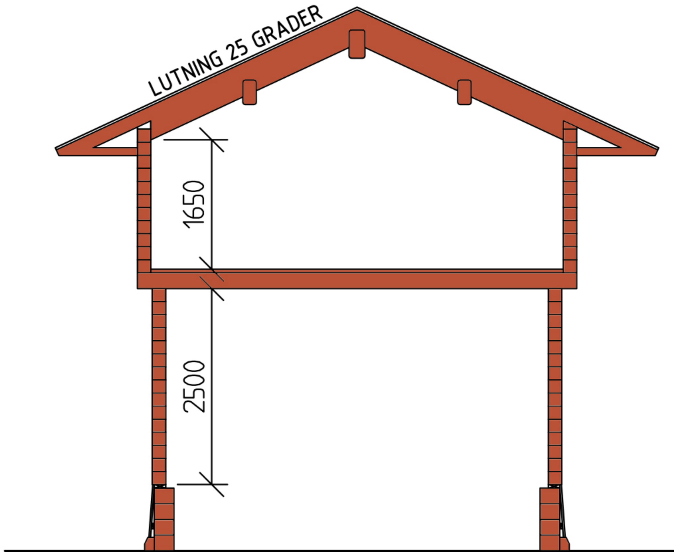
PRINCIPSEKTION
