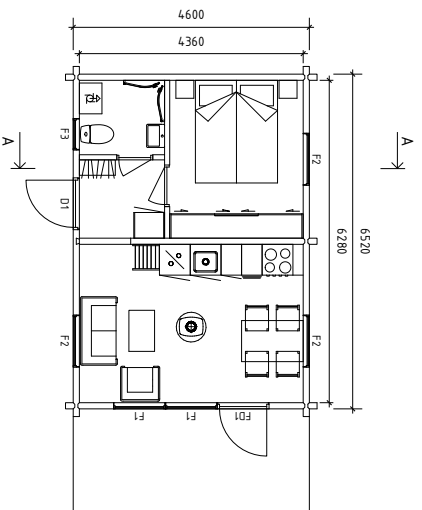
BOTTEPLAN 1:100 (A3)
