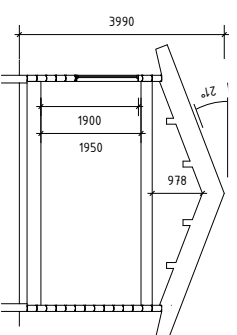
SEKTION A-A (PLINT/TORPARGRUND) 1:100 (A3)
