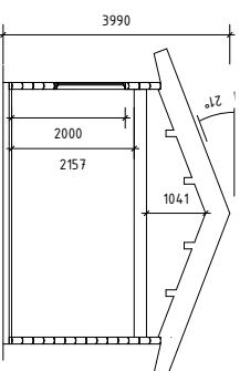
SEKTION A-A (PLATTÅ PÅ MARK) 1:100 (A3)
