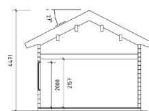
SEKTION A-A (PLATTA PÅ MARK) 1:100 (A3)
