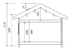
SEKTION A-A (PLINT/TORPARGRUND) 1:100 (A3)
