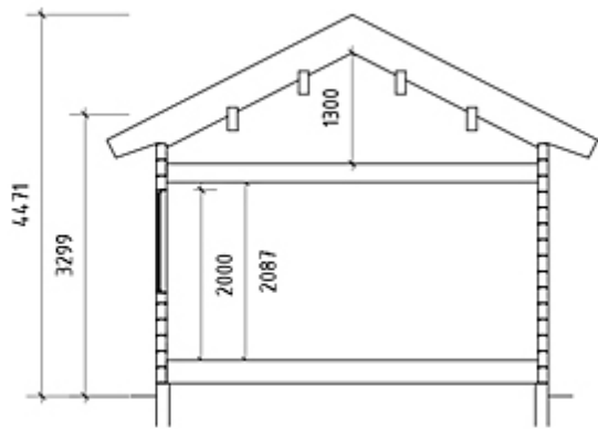
SEKTION A-A (PLINT/TORPARGRUND)
