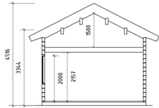
SEKTION A-A (PLATTA PÅ MARK)
